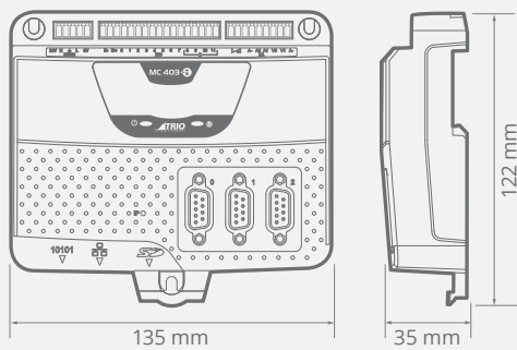
Wymiary - MC403-X
